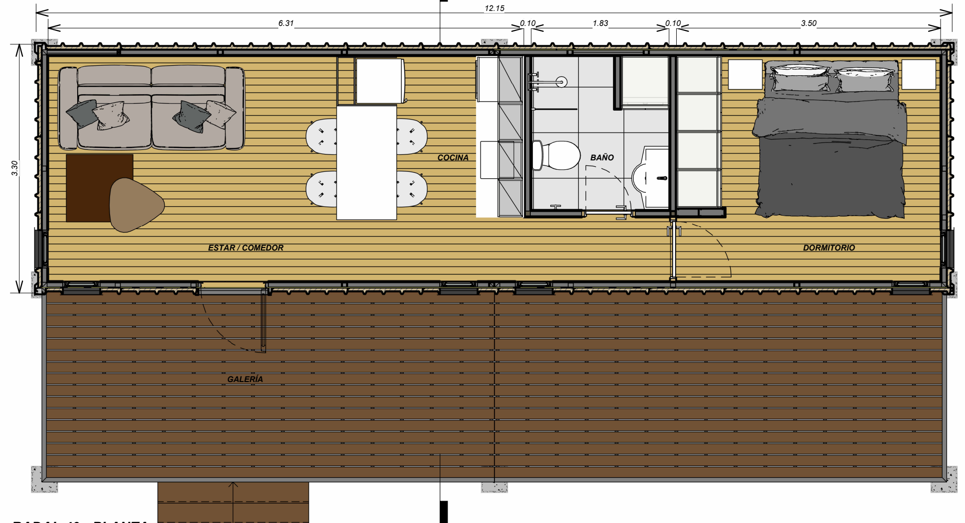
RADAL 40 - PLANTA 1 : 50
