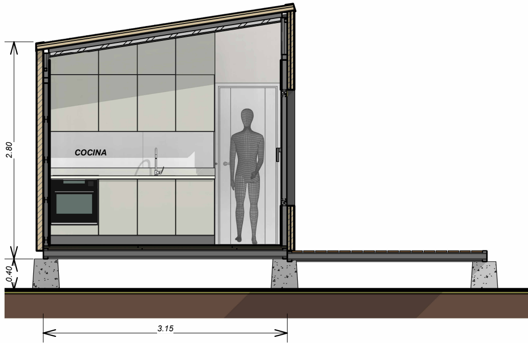
SECCIÓN - COCINA 1 : 50
